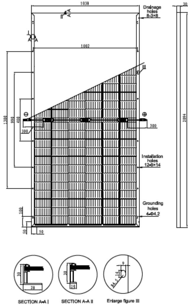
Figure 2. Figure@144HDF unit: mm 图 2 示意图@144HDF 单位 : mm
