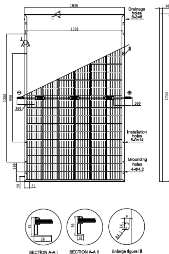
Figure 1. Figure@120HDF unit: mm 图 1 示意图@120HDF 单位：mm
